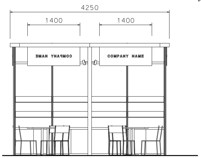
ELEVATION - B
