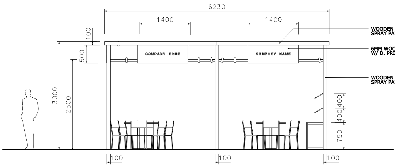
ELEVATION - A
