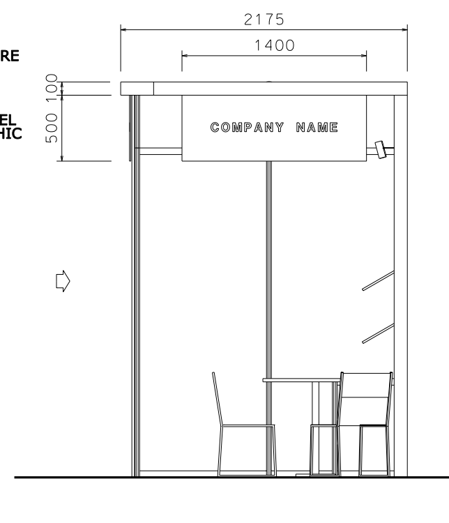
ELEVATION - B
