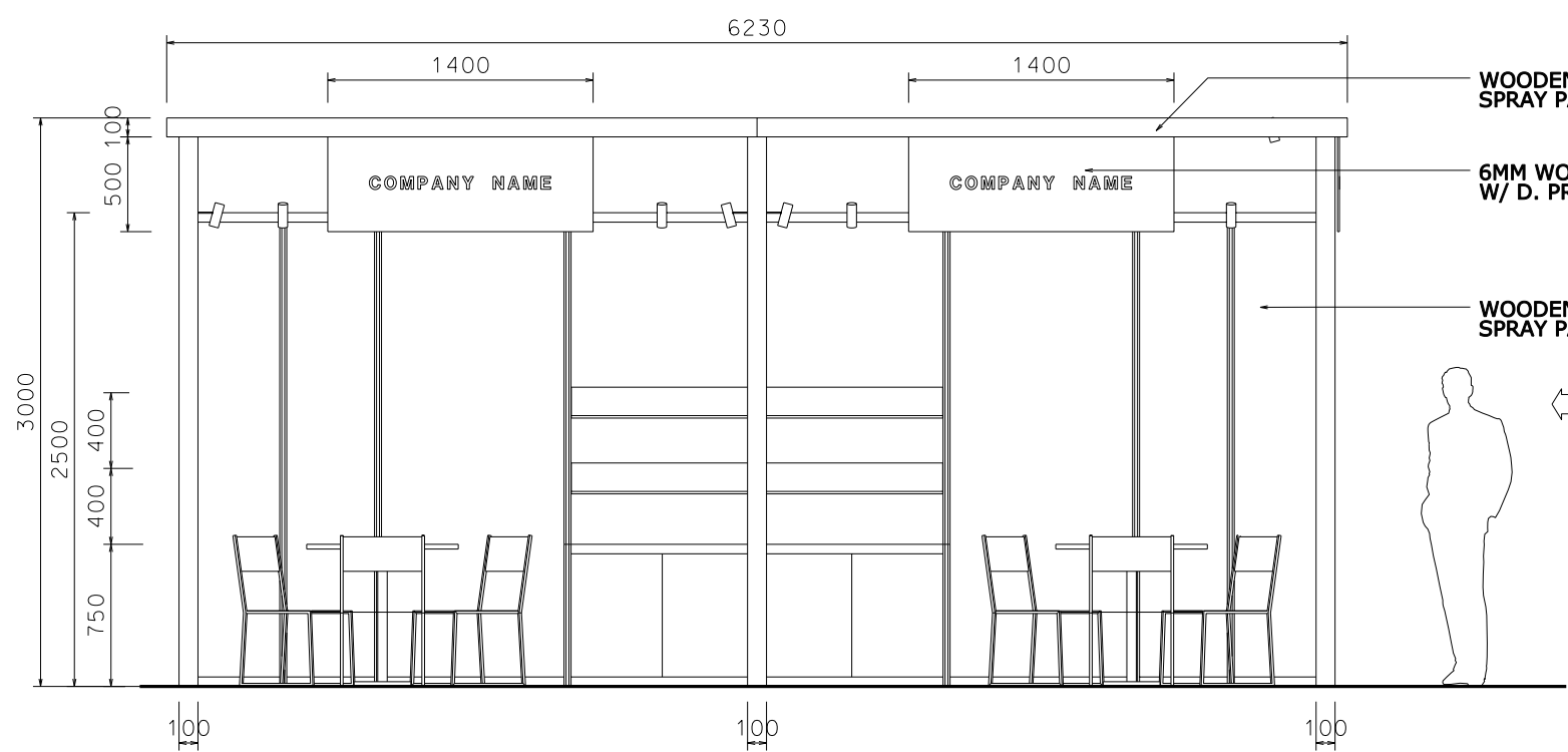
ELEVATION - A
