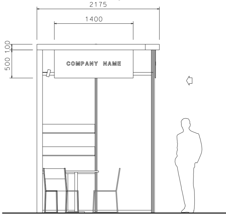
ELEVATION - B
