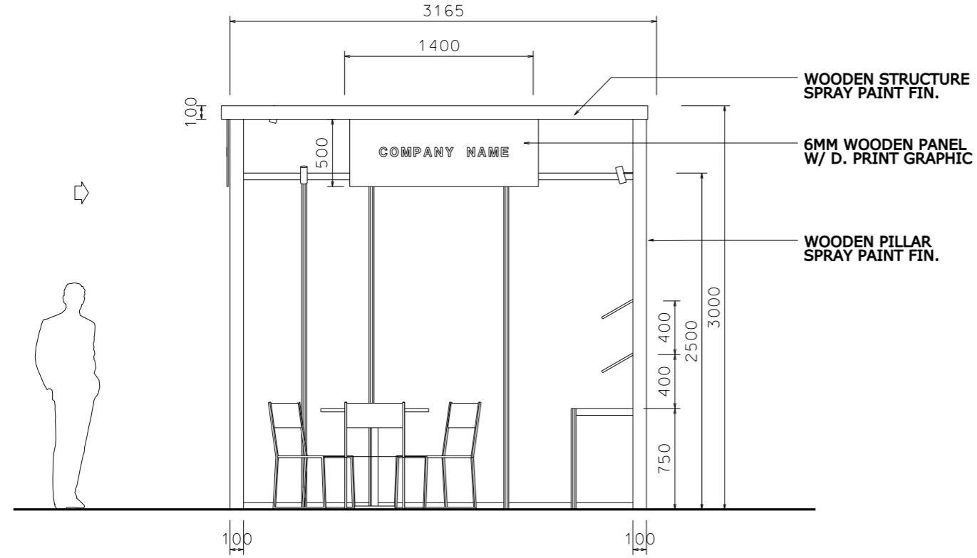
ELEVATION - A
