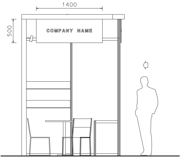
ELEVATION - B
