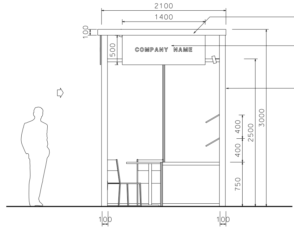
ELEVATION - A
