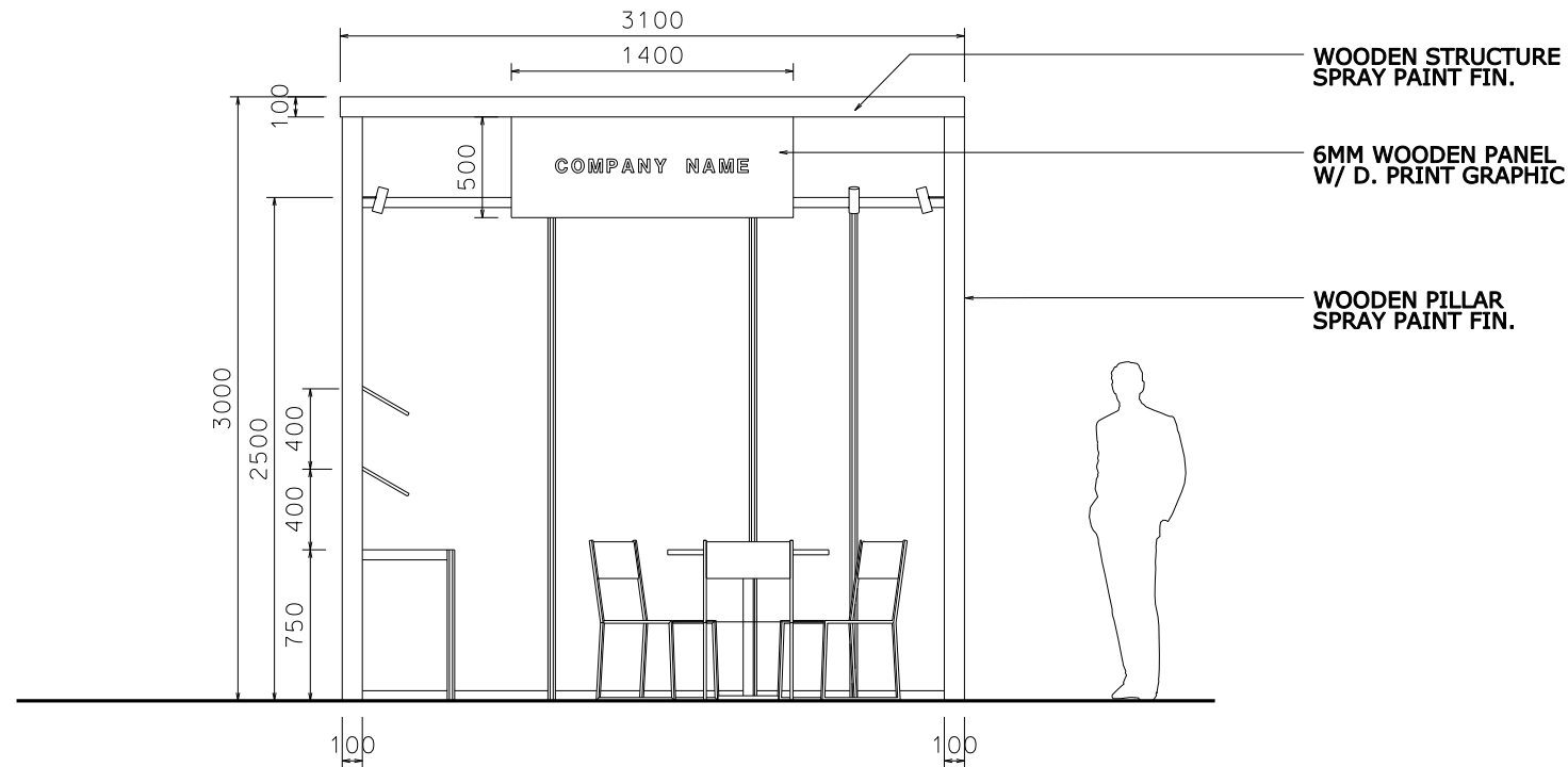
ELEVATION - A
