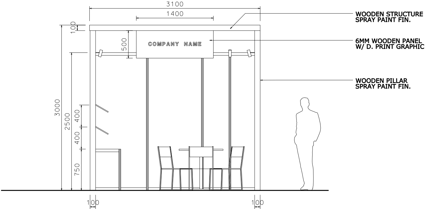
ELEVATION - A
